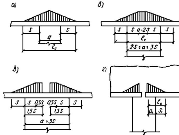
Рис. 15. Распределение давления в кладке над опорами висячих стен
