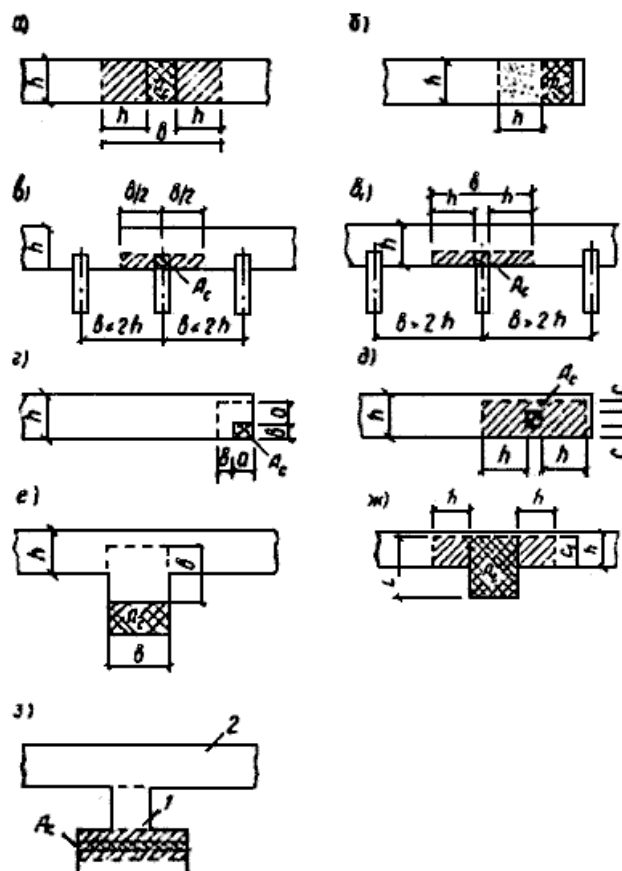
Рис. 9. Определение расчетных площадей сечений при местном сжатии а — ж — различные случаи местного сжатия
