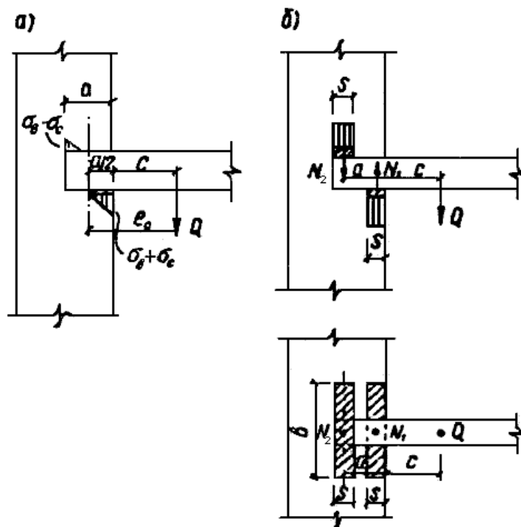
Рис. 14. Расчетные схемы заделки консольных балок
