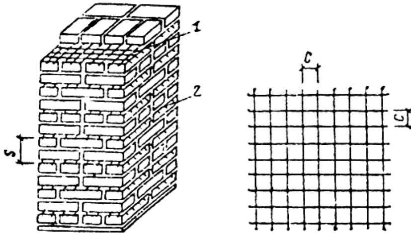
Рис. 10. Поперечное (сетчатое) армирование каменных конструкций
