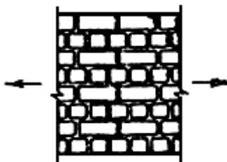
Рис. 2. Растяжение кладки по перевязанному сечению
