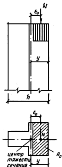
Рис. 5. Внецентренное сжатие
