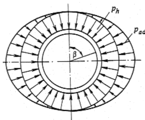
Черт. 5. Схема распределения основного p_h и дополнительного p_{ad} горизонтального давления
