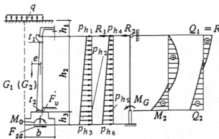
Черт. 3. Расчетная схема стены подвала
