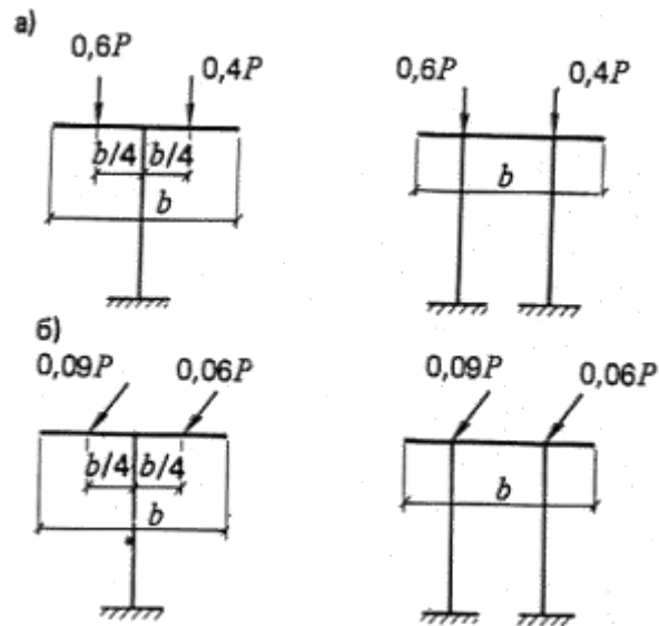
Черт. 9. Распределение нагрузки при расчете колонн и фундаментов промежуточных отдельно стоящих опор по поперечному сечению трассы а - схема распределения вертикальной нагрузки; б - то же, горизонтальной нагрузки; P = pb - нормативная вертикальная нагрузка на опору или на соответствующий ярус опоры, где p - нормативное значение интенсивности вертикальной нагрузки на траверсу, определяемое по формуле (51)
