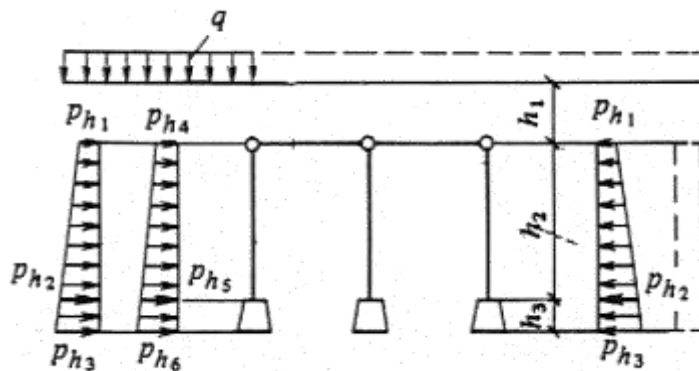
Черт. 2. Расчетная схема поперечной рамы подвала
