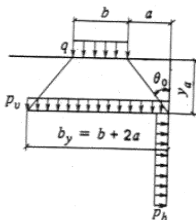
Черт. 2. Схема распределения давления от полосовой нагрузки
