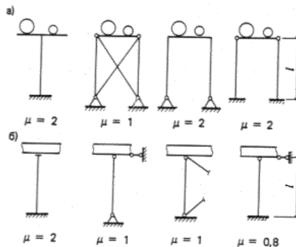
Черт. 10. Значения коэффициентов для определения расчетных длин l_0 = \mu l колонн опор а - в плоскости, перпендикулярной оси трубопроводов; б - в плоскости оси трубопроводов
