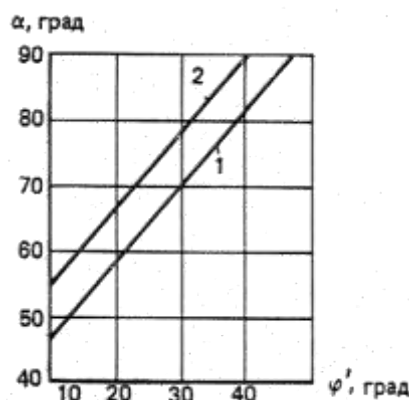
Черт. 6. Графики для определения угла наклона стенок бункеров для связных материалов 1 - для бункеров с прямоугольной формой выпускного отверстия (отношение сторон 3:1 и более); 2 - для воронок конической формы с круглым отверстием или пирамидальной формы с квадратным отверстием; \varphi - угол трения сыпучего материала по стенкам бункера; \alpha - угол наклона стенки к горизонтали
