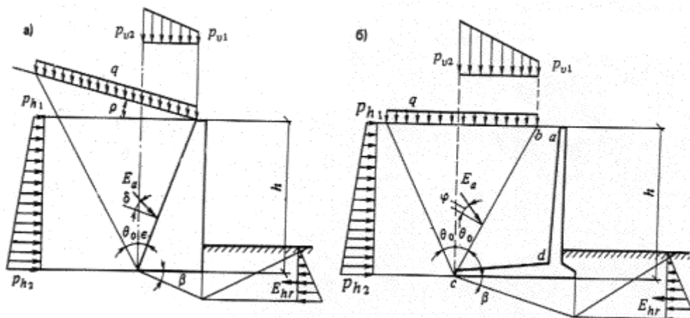
Черт. 1. Расчетные схемы подпорных стен а - массивных; б - углового профиля
