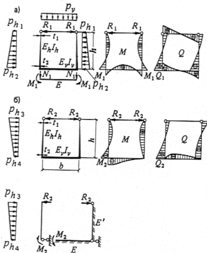
Черт. 4. Расчетная схема тоннеля с шарнирами в уровне плит перекрытия а - симметричное нагружение; б - одностороннее нагружение
