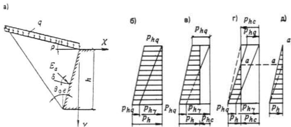
Черт. 1. Схема давления грунта
