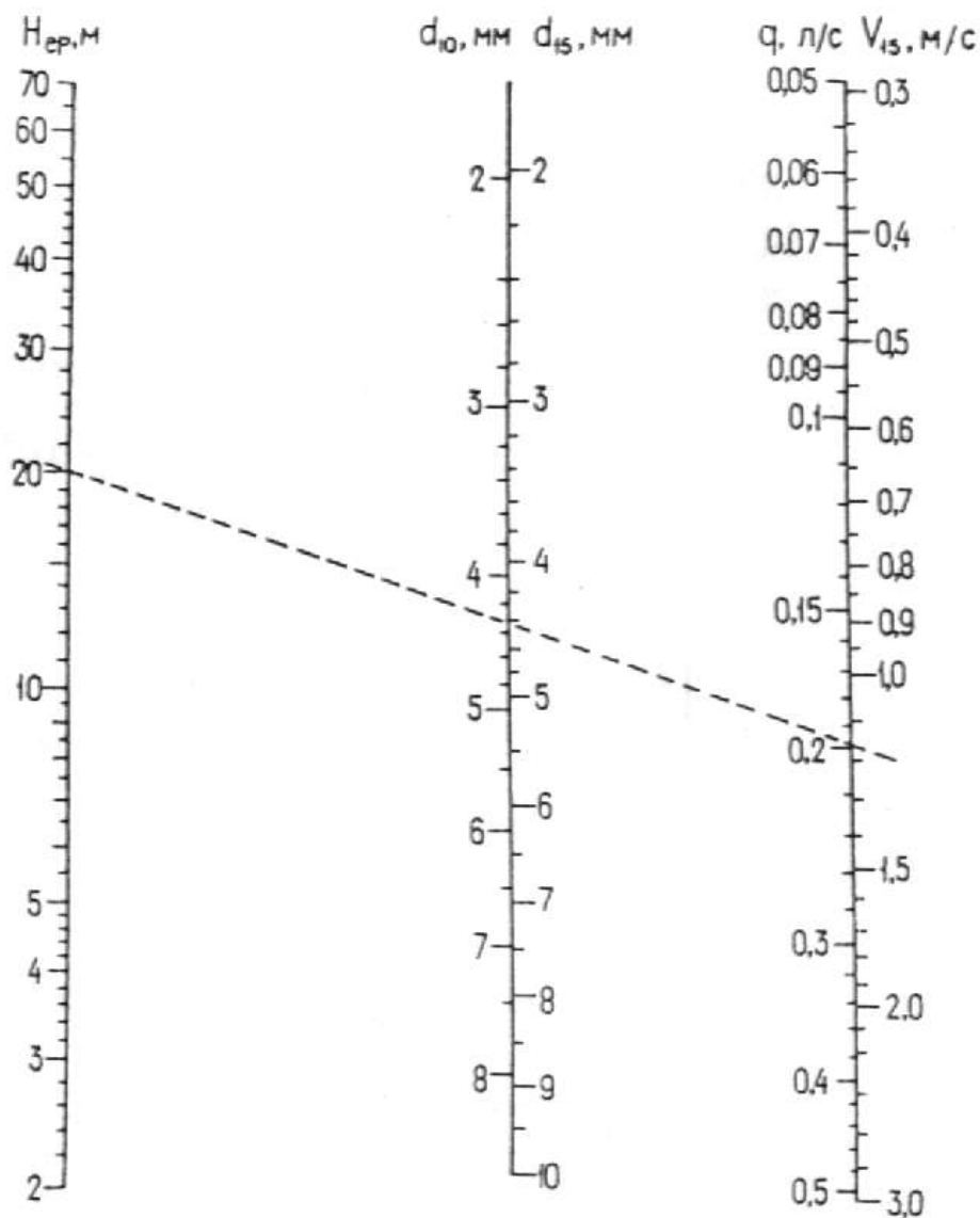
Черт. 6. Номограмма для определения отверстий диафрагм, устанавливаемых у смесителей водоразборной арматуры санитарных приборов d_{10} ( d_{15} ) — диаметр отверстия диафрагмы, мм, устанавливаемой в соединительных патрубках (подводках) смесительной водоразборной арматуры с условным проходом d = 10 и 15 мм; v_{15} — скорость движения воды, м/с, в подводке d = 15 мм
