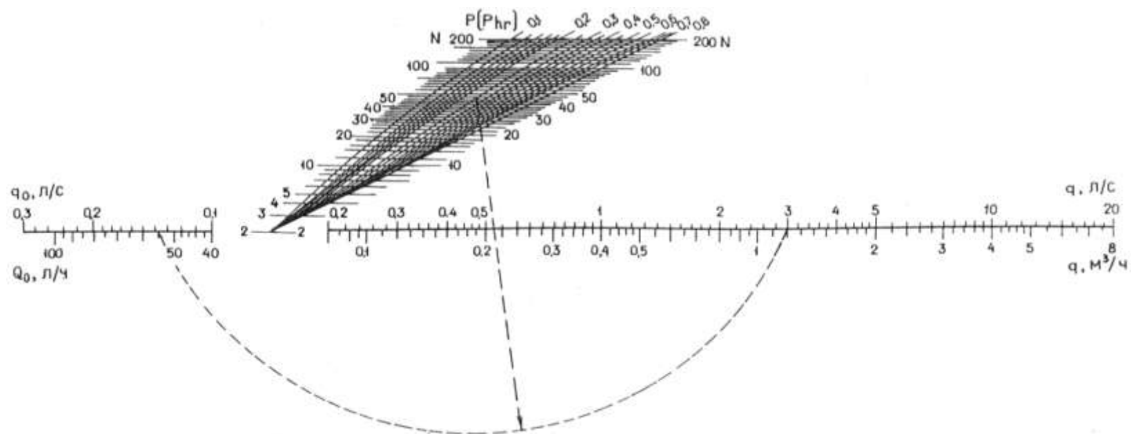
Черт. 3. Номограмма для определения секундных и часовых расходов воды q при q_0 \leq 0,3 \text{ л/с} , N \leq 200 и P > 0,1
