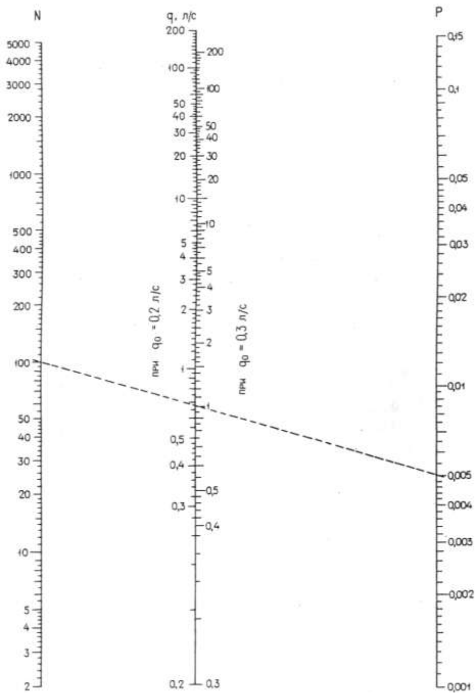
Черт. 2. Номограмма для определения секундных расходов воды q при q_0 = 0,2 и 0,3 \text{ л/с} и P \leq 0,15
