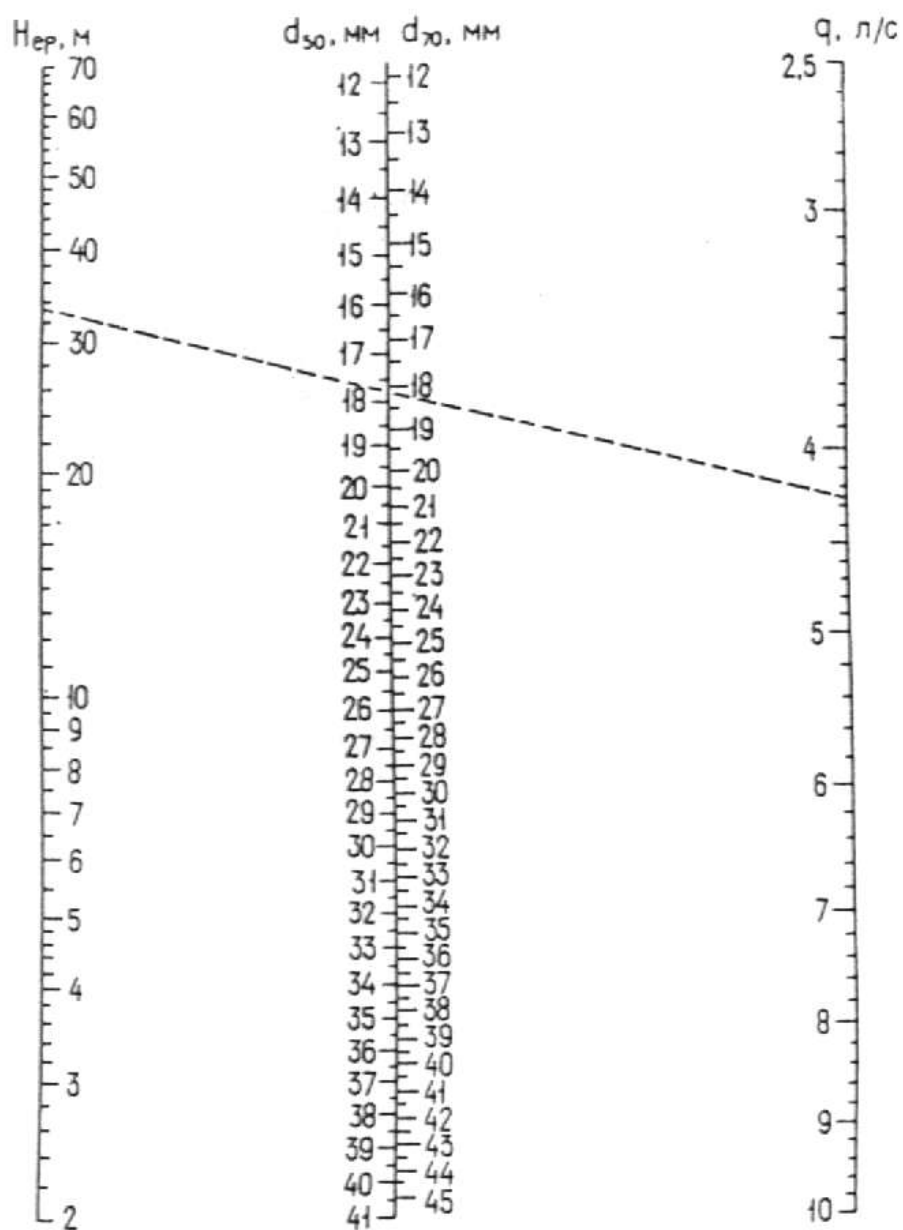
Черт. 5. Номограмма для определения диаметров отверстий диафрагм, устанавливаемых между соединительными головками и пожарными кранами d_{50} — диаметр отверстия диафрагмы, устанавливаемой у пожарного крана диаметром 50 мм; d_{70} — то же, диаметром 70 мм
