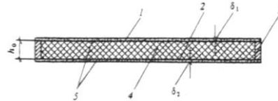
Черт.5. Поперечное сечение бескаркасной панели с обрамлением
