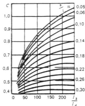
Черт.6. График для определения коэффициента C
