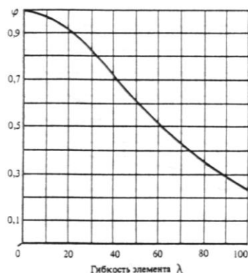
Черт.10. График определения коэффициента продольного изгиба \varphi .
