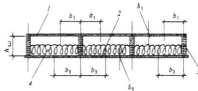
Черт.2. Поперечное сечение каркасной плиты
